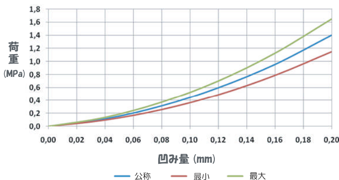
Compressibility curve : 圧縮曲線
